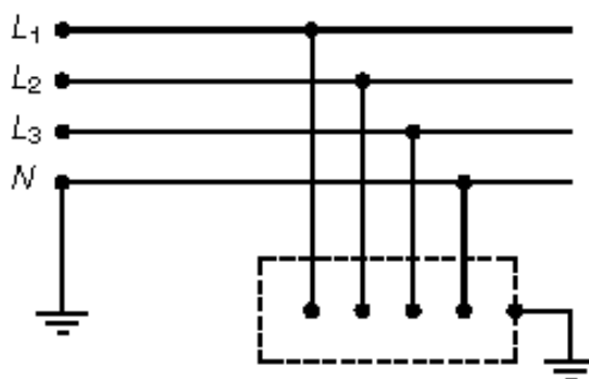
Sistema TT
