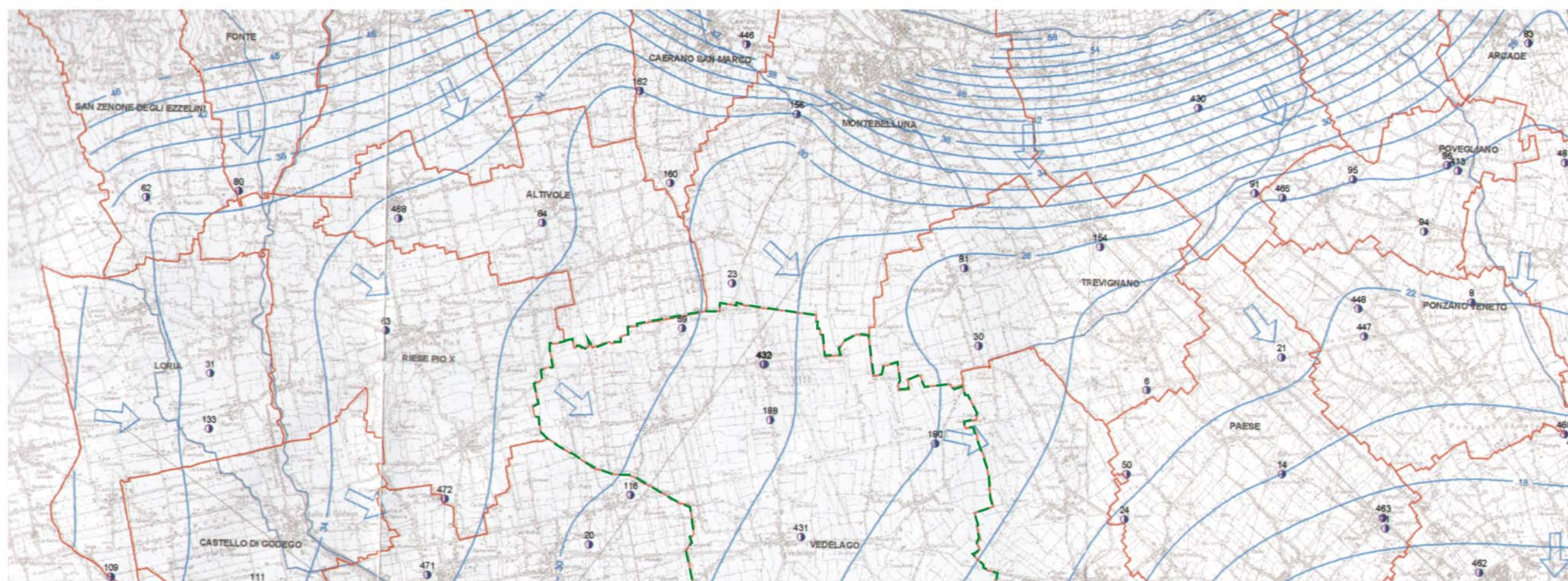
FIG. 7 - CARTA IDROGEOLOGICA GENERALE (1)
