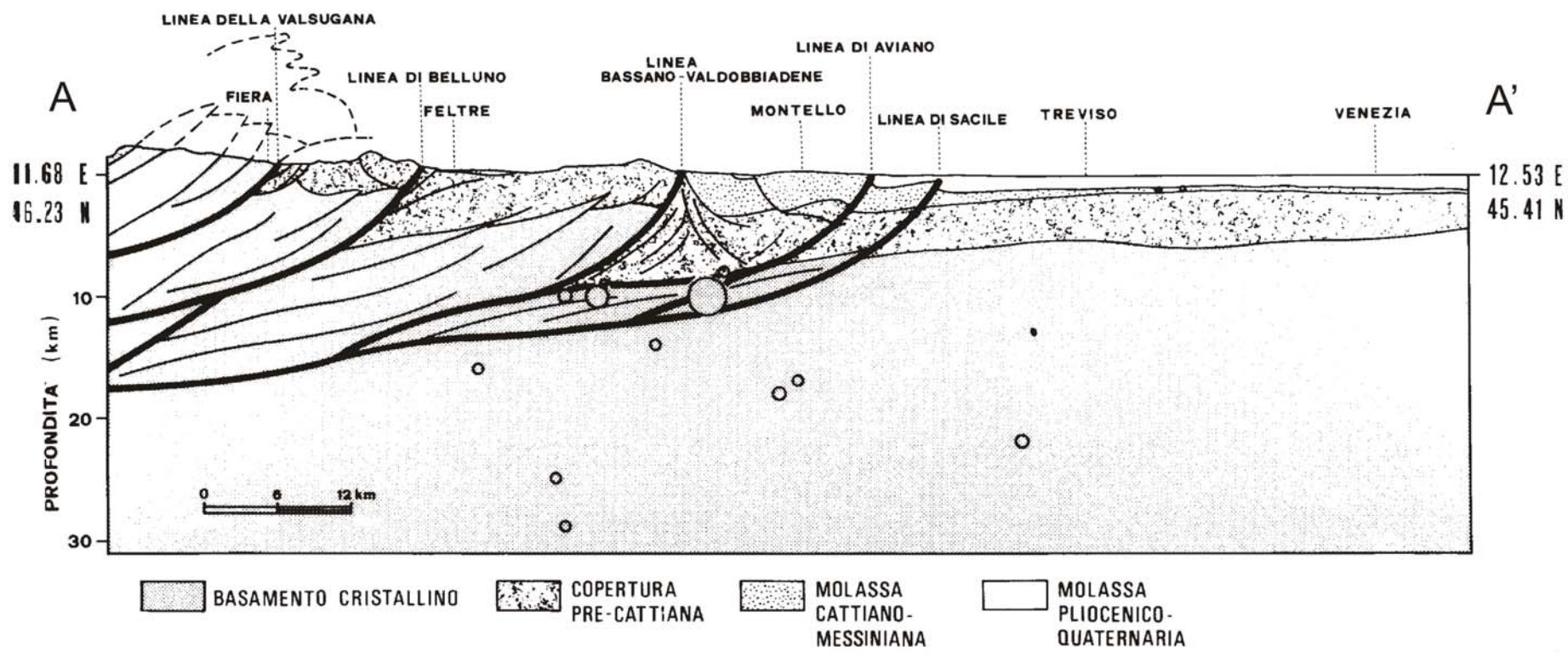
FIG. 4 - SEZIONE GEOLOGICA E GEOFISICA DELLA ZONA IN ESAME (la traccia è riportata in FIG. 5 - Gli ipocentri segnati sono relativi ai terremoti avvenuti nel periodo 1966÷1984) (da AA.VV. "Modello sismotettonico dell'Italia Nord Orientale", CNR-GNDT, Rendiconto 1, Trieste 1987)
