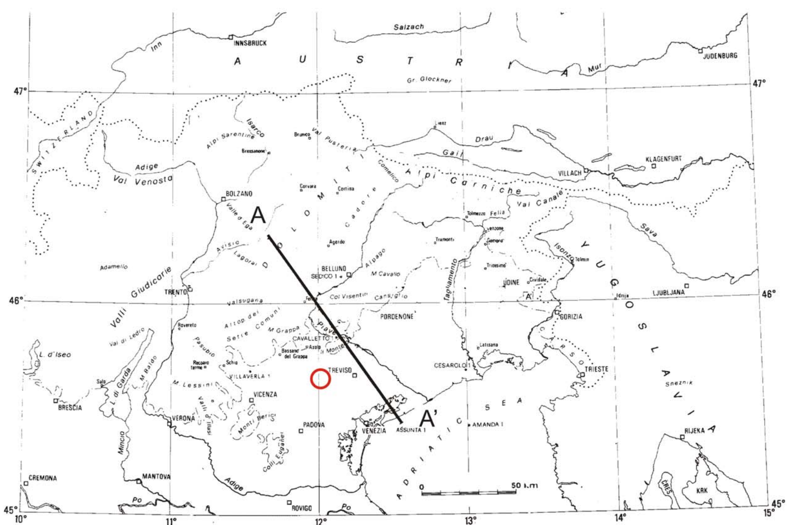
FIG. 5 - LOCALIZZAZIONE DELLA SEZIONE GEOLOGICA E GEOFISICA RIPORTATA IN FIG. 4 (v. in neretto la traccia della sezione denominata A-A') (da AA.VV. "Modello sismotettonico dell'Italia Nord Orientale", CNR-GNDT, Rendiconto 1, Trieste 1987) ○ Comune di Veduggio
